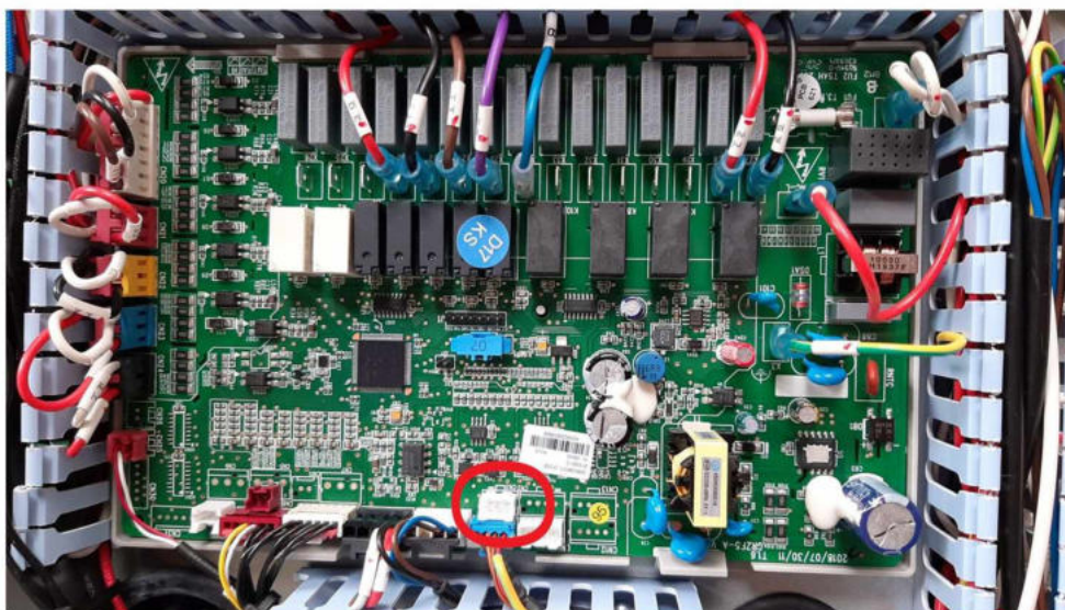
Jednostka wewnętrzna pompa ciepła Versati III
