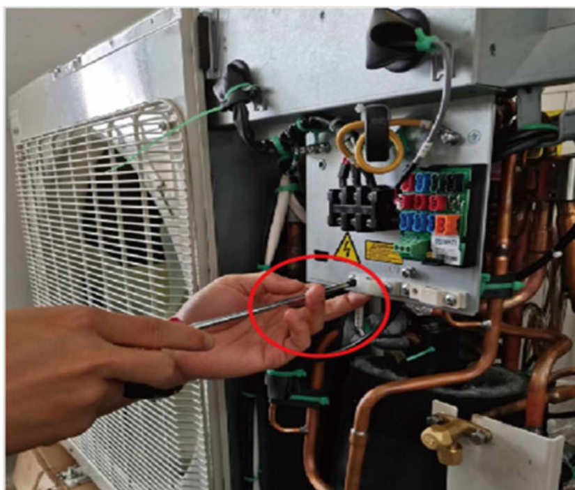
Odkręcanie obejmy zaciskowej przewodów jednostki zewnętrznej
