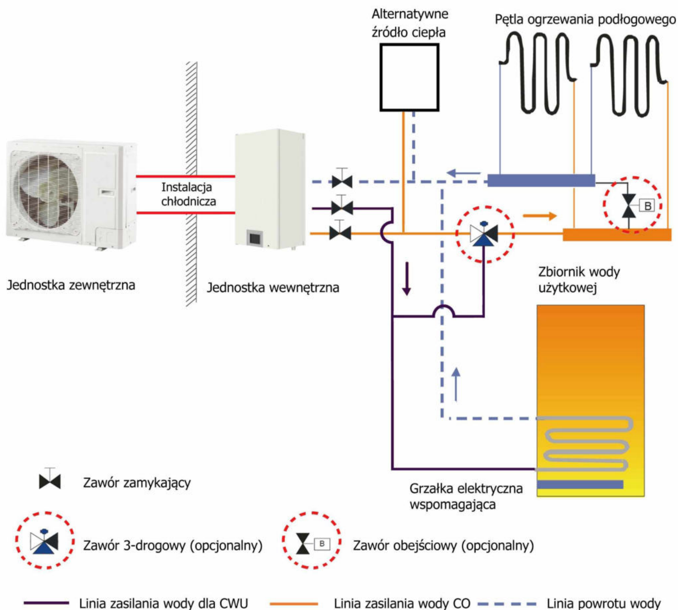
Przykład 4: Podłączenie zasobnika wody użytkowej, pętli ogrzewania podłogowego oraz alternatywnego źródła ciepła.
