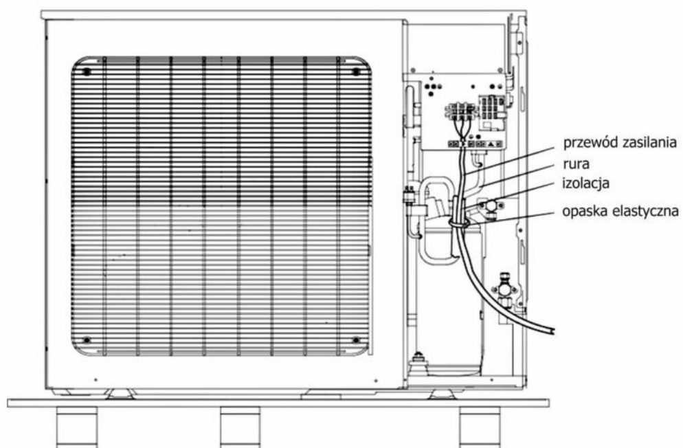
Schemat prowadzenia i podłączenia przewodów zasilania
