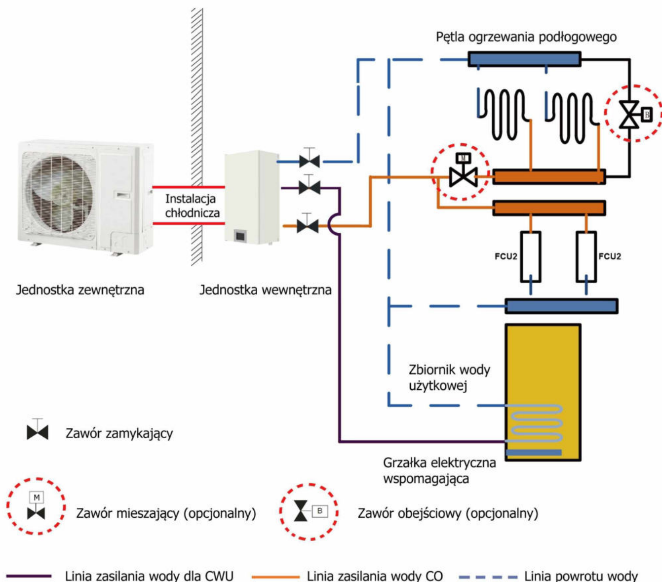
Przykład 3: Podłączenie zasobnika wody użytkowej, pętli ogrzewania podłogowego i klimakonwektorów FCU
