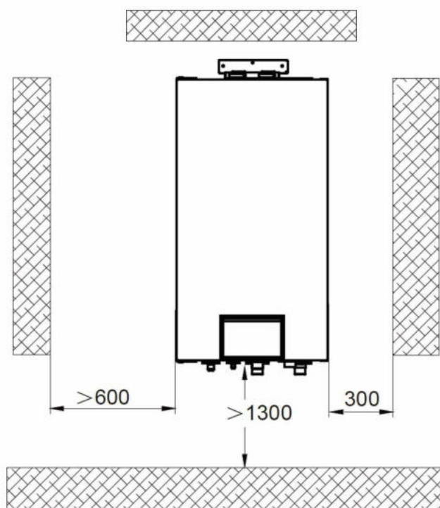
Przestrzeń serwisowa
