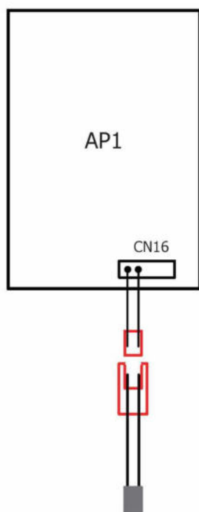
Opcjonalny czujnik temperatury wody
